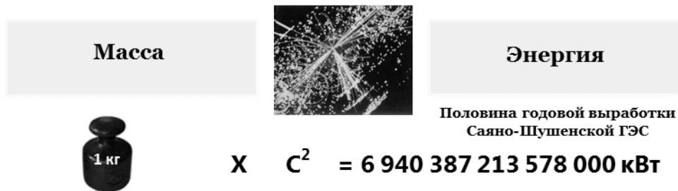
Рис. 10. Бозонный уровень энергии
