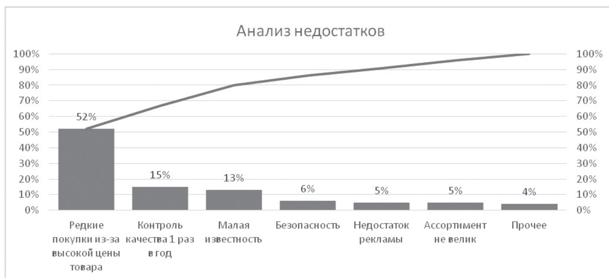
Рисунок 1. Диаграмма Парето
